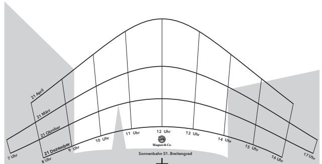
Bild 5 Die Gebäude- und Baumrisse können Sie auf die Sonnenbahnfolie oder auf eine zweite dahintergeklebte Folie mit einem wasserlöslichen Foliestift aufzeichnen.
