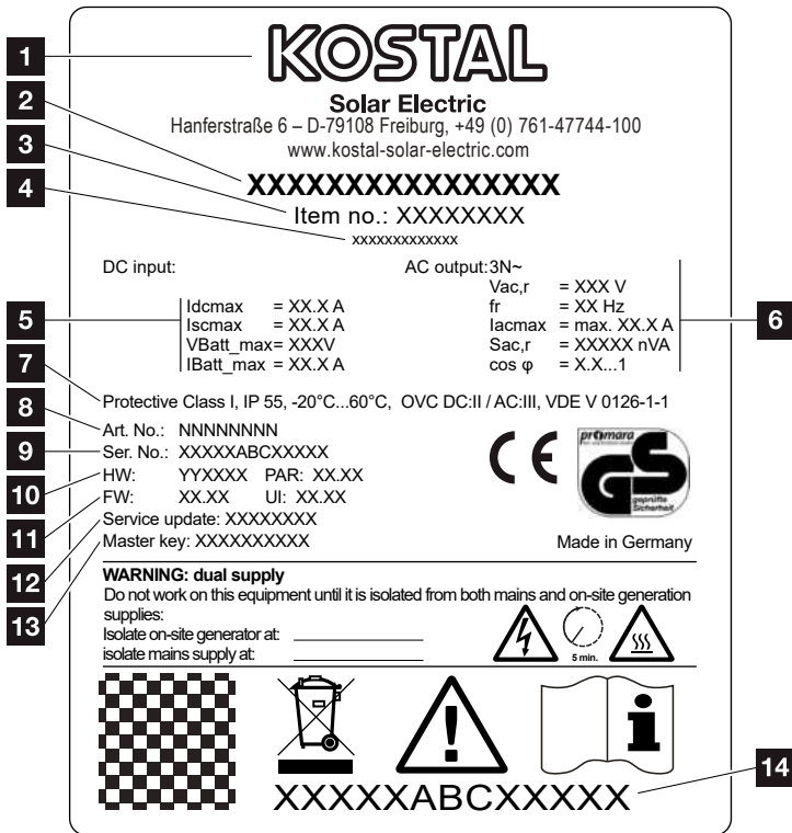
Abb. 58: Typenschild
