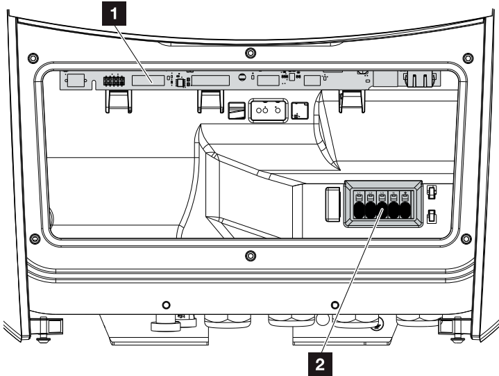
Abb. 11: Speicherwechselrichter (Innenansicht)
