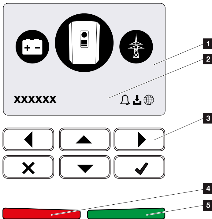
Abb. 12: Bedienfeld
