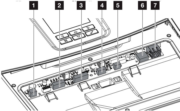
Speicherwechselrichter (Innenansicht)
