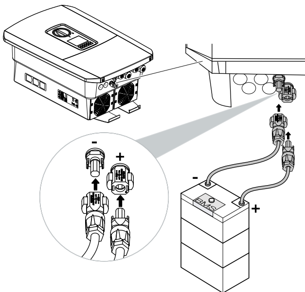
Abb. 32: DC-Anschluss Batterie
