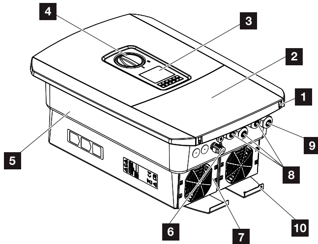
Abb. 8: Speicherwechselrichter (Außenansicht)
