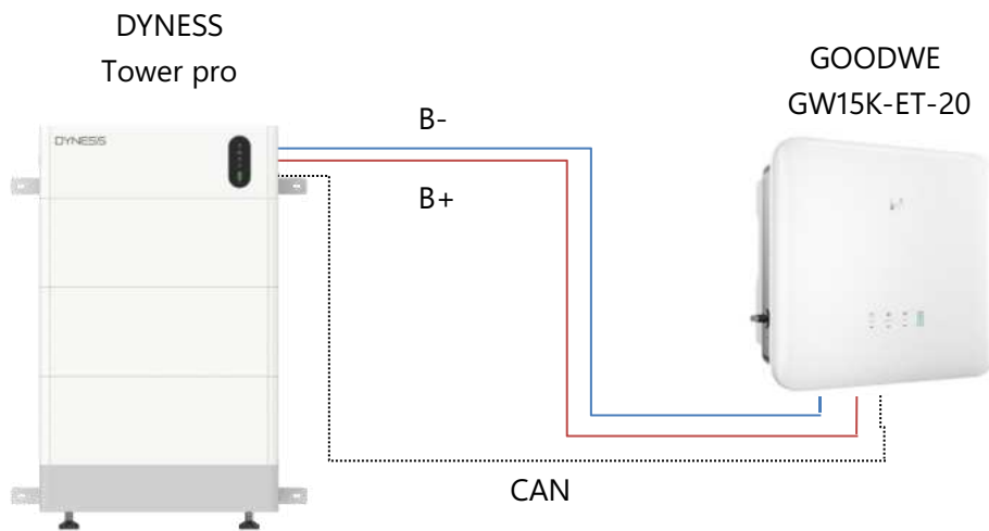
Anschlussplan von Tower pro und GOODWE
