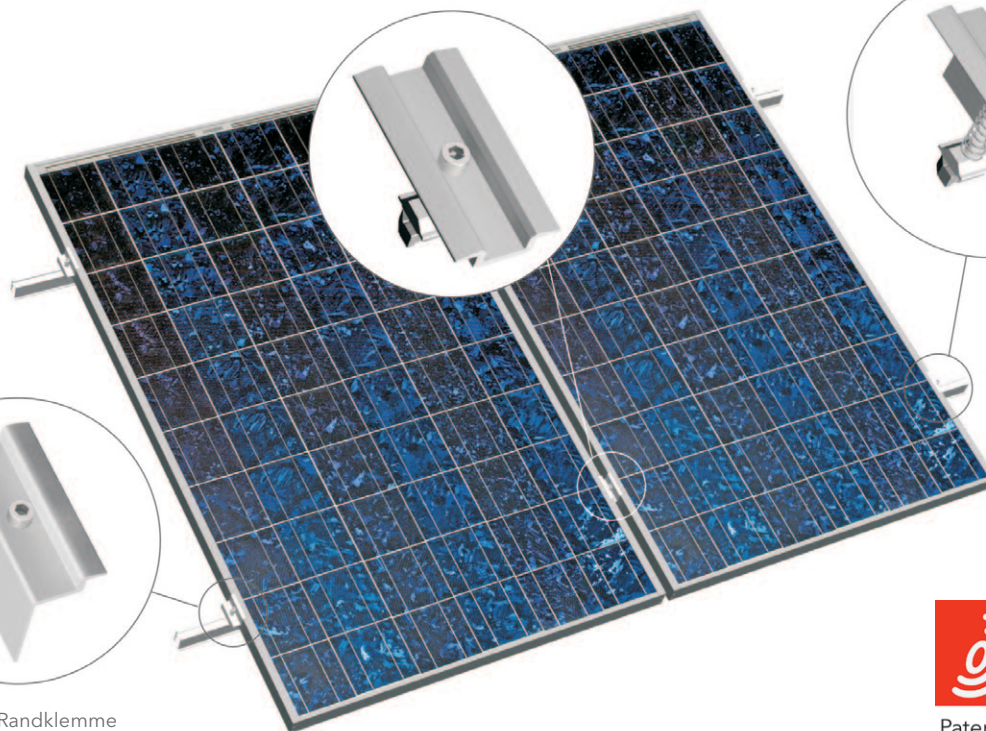
TRIC clip Mittelklemme
