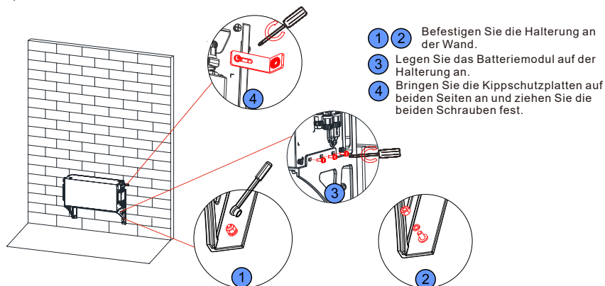
Abbildung 4-10: Befestigung der Halterung an der Wand
