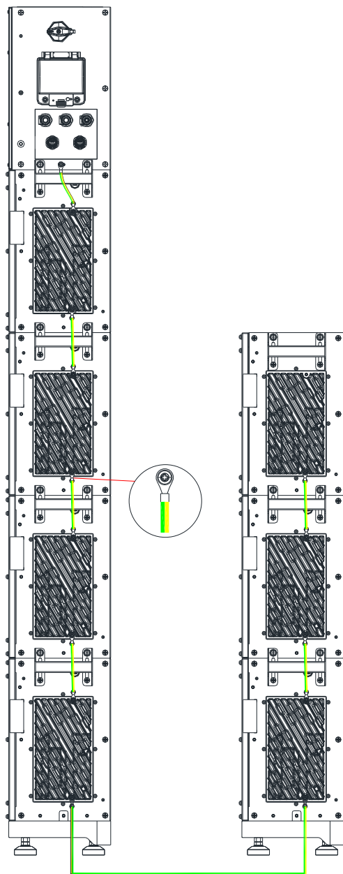
Abbildung 4-23: Zweireihige Montage
