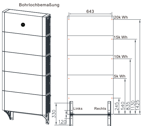
Abbildung 4-7: Bohrlochbemaßung
