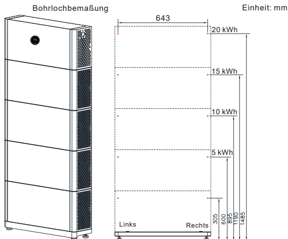
Abbildung 4-14: Bohrlochbemaßung
