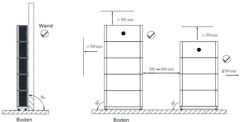
Abbildung 4-2: Standmontage
