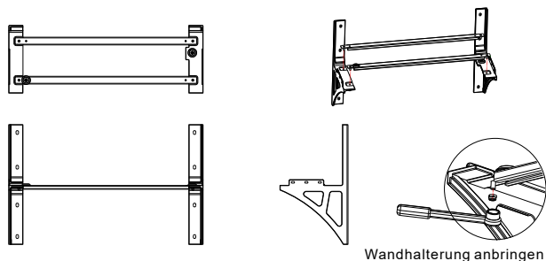
Abbildung 4-8: Wandhalterung anbringen
