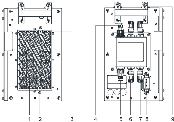
Abbildung 1-5: Anschlüsse vom Batteriemodul
