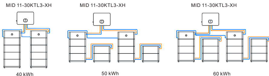
Abbildung 4-21: Montageplan des Batteriesystems mit einer Kapazität von 40 kWh bis 60 kWh
