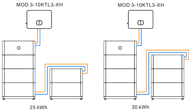
Abbildung 4-20: Montageplan des Batteriesystems mit einer Kapazität von 25 kWh bis 30 kWh
