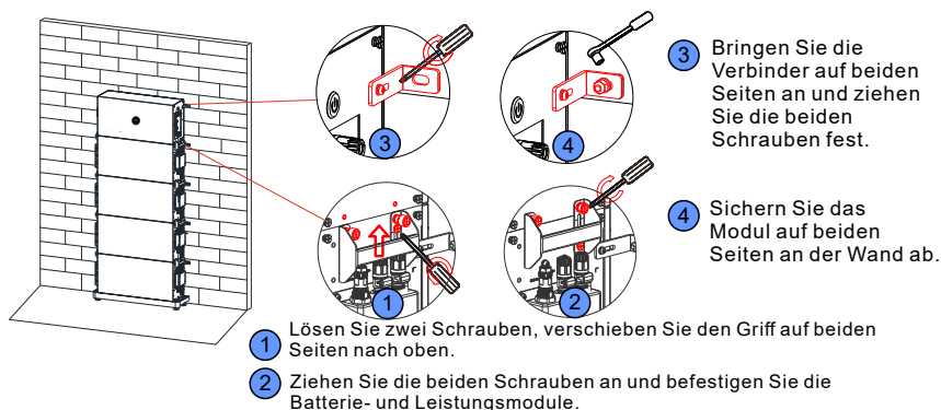
Abbildung 4-18: Montage des Leistungsmoduls
