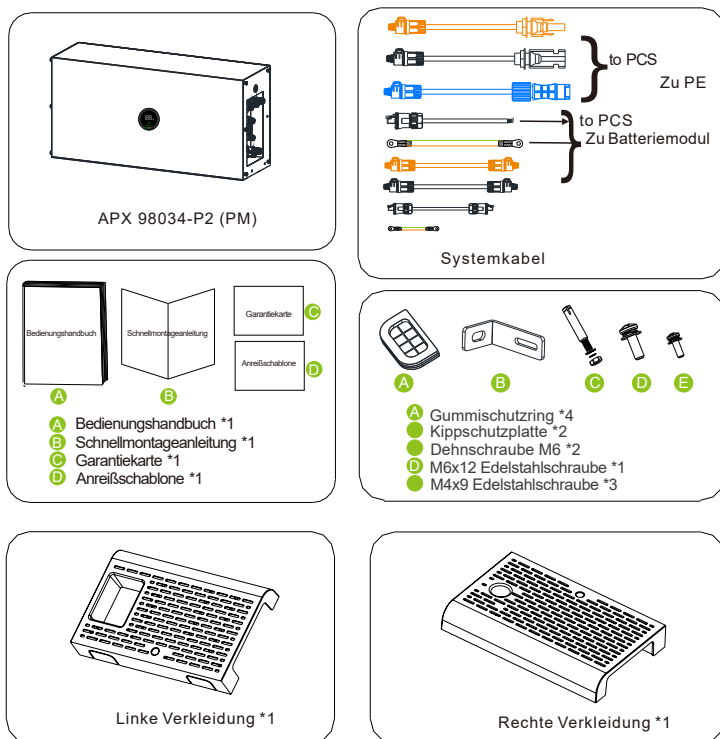
Abbildung 4-5: Komponenten des APX 98034-P2
