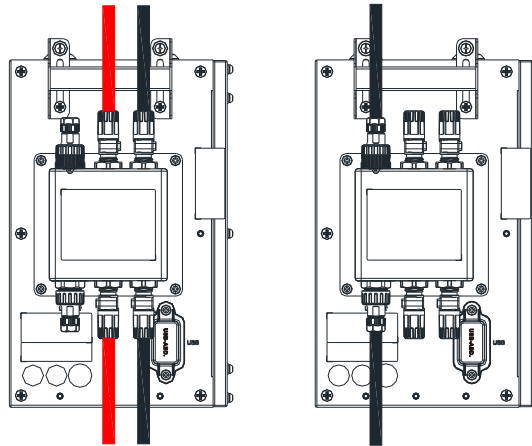
Abbildung 4-25: Anschlussdiagramm APX 5.0P-B1
