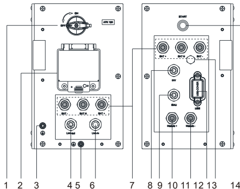
Abbildung 1-2: Anschlüsse des Leistungsmoduls
