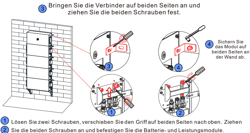
Abbildung 4-13: Montage des Leistungsmoduls
