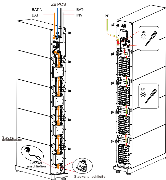
Abbildung 4-22: Einreihige Montage
