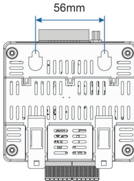
Abbildung 4-1 Befestigungsöffnungen
