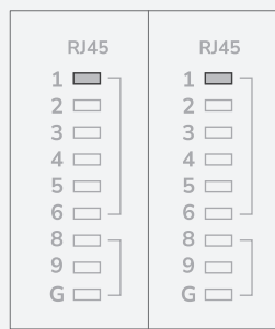
Ideale Verbindung
