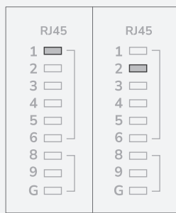
Falscher Verdrahtungsstandard
