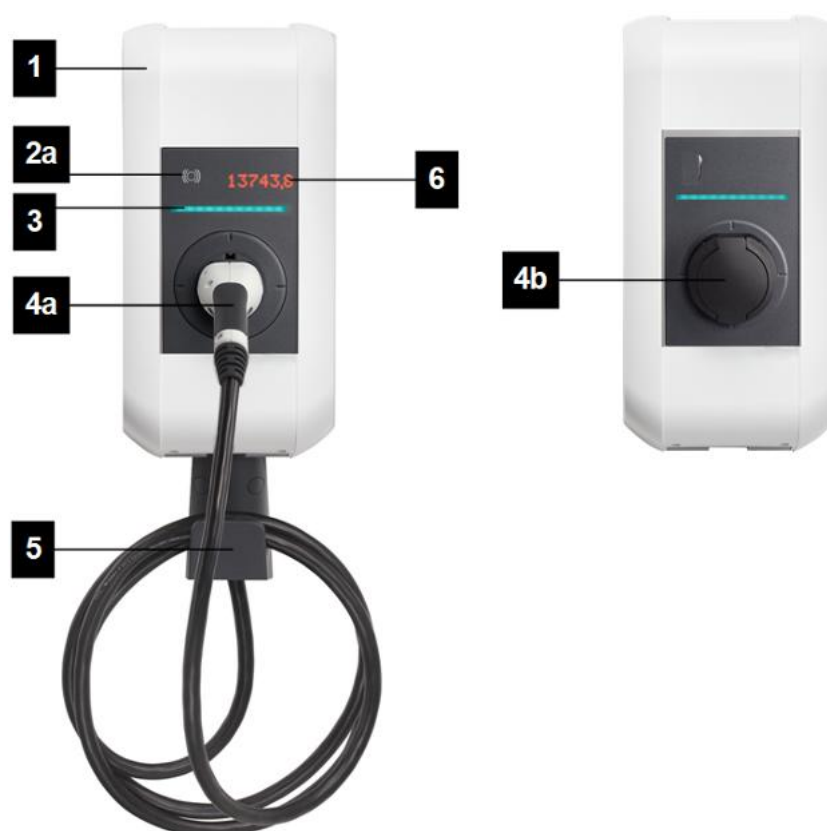
Abb. 4-4: Übersicht Ladestation
