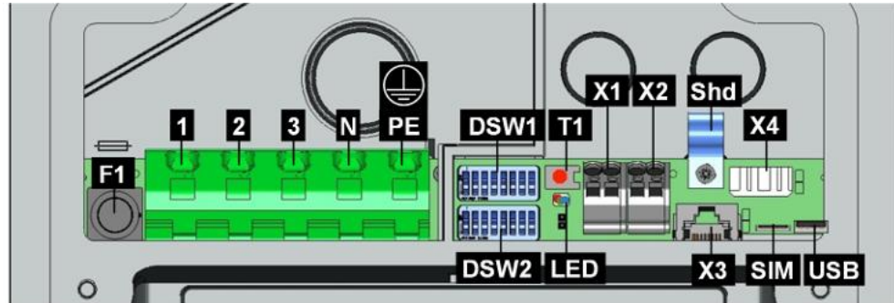
Abb. 7-16: Anschlussübersicht
