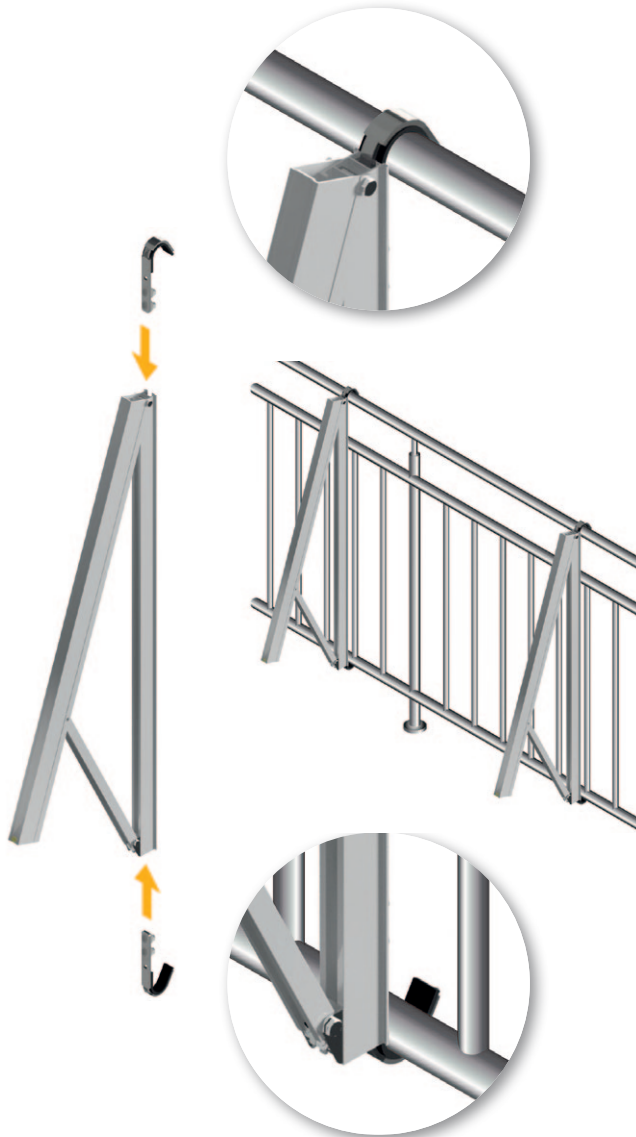
TRIC Balcony mit Montagesystem TRIC F Fassade
